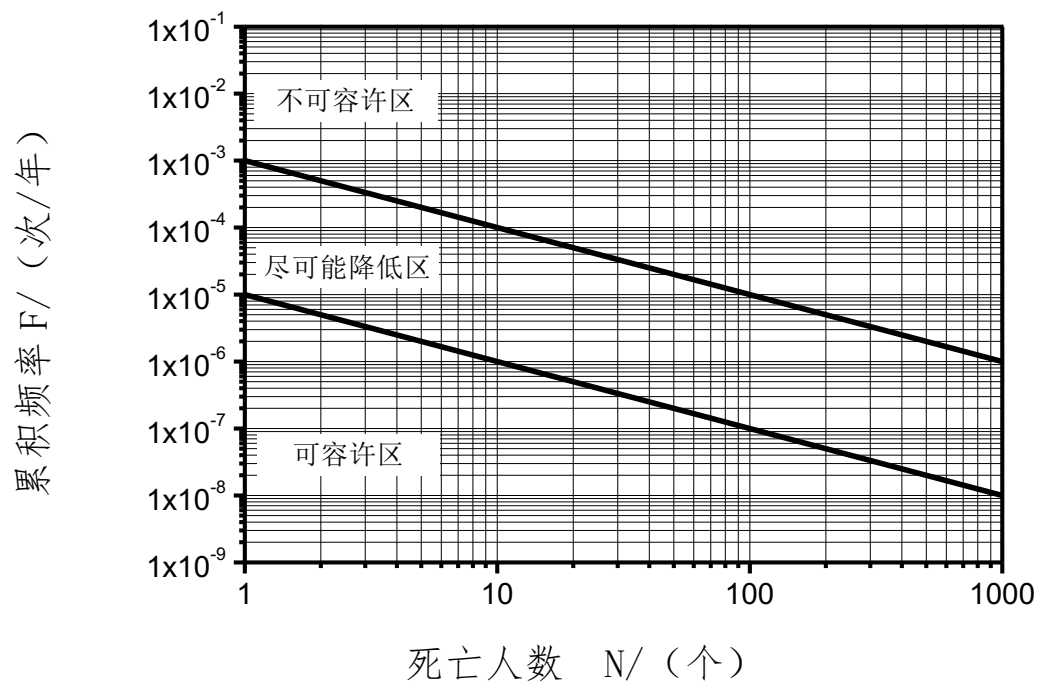
图 1 可容许社会风险标准 ( F-N ) 曲线
